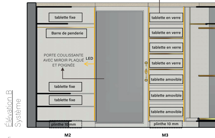
Détail M3 Vue isométrique
