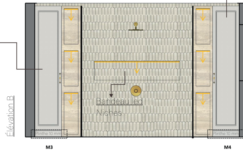
Élévation B Détail M3 -M4
