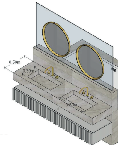
Élévation C Détail M5
