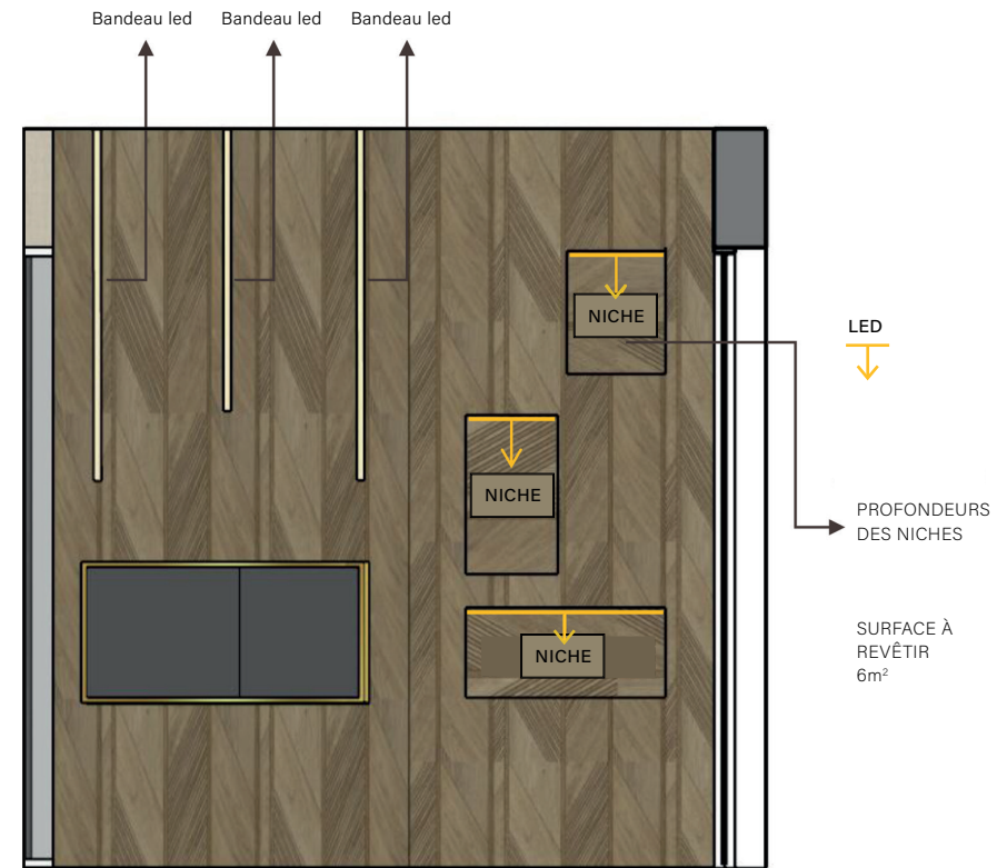
Élévation D Vue avec textures
